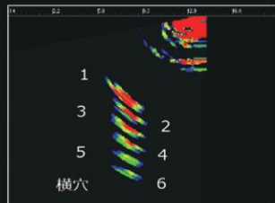
近接欠陥画像例 (横穴Φ1mm間隔0.1mm)
