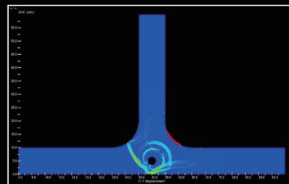
隅肉溶接検査シミュレーション
