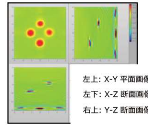
検出結果画像 欠陥寸法:Φ0.7×d2およびd3
